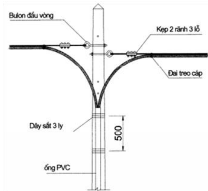
Hình C.2. Kết cuối dây treo cáp ở nơi cáp vào và ra tủ
