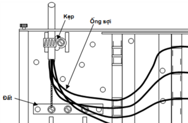
Hình C.9 - Lắp đặt kẹp cáp
