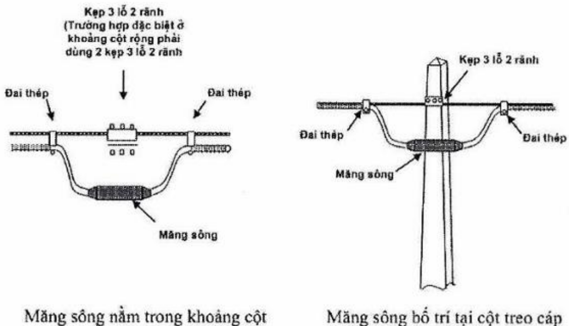
Hình C.4 - Măng sông cáp treo
