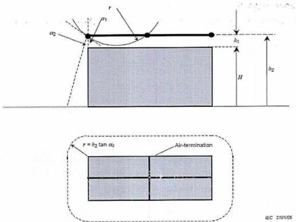
Hình B.4 - Vùng được bảo vệ bởi các dây dẫn dạng lưới tách biệt, xác định theo phương pháp góc bảo vệ và phương pháp quả cầu lăn
