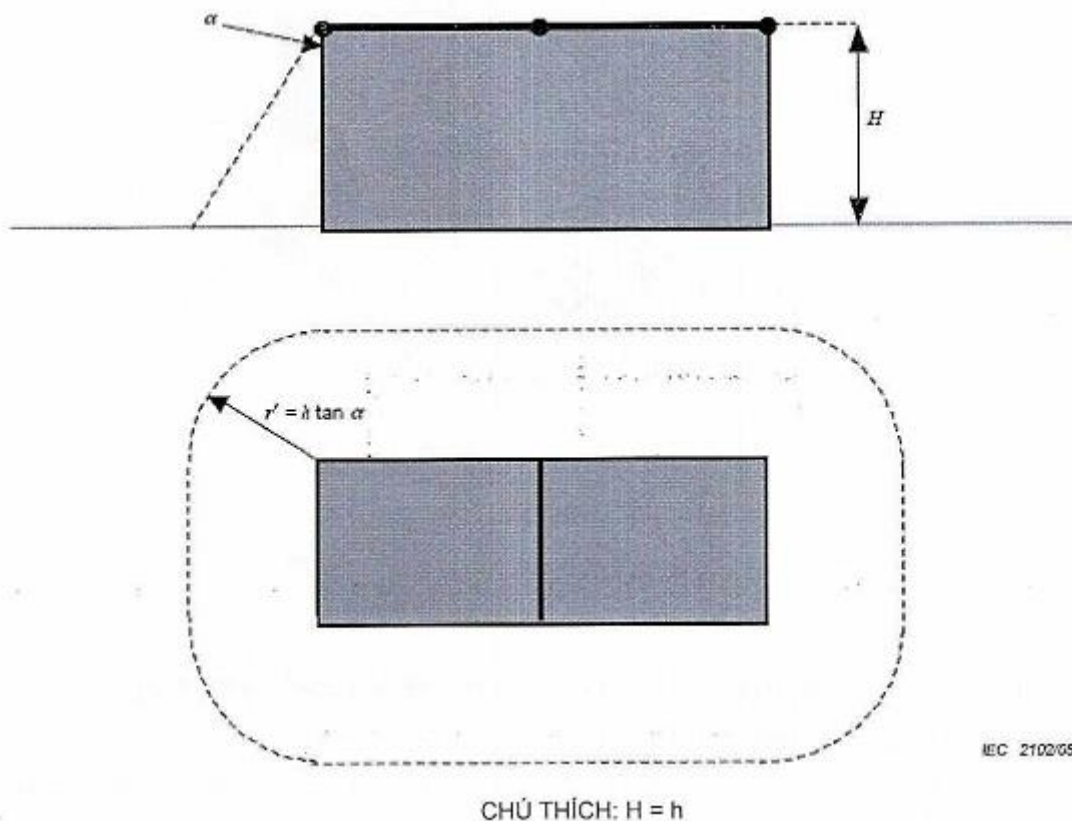
Hình B.5 - Vùng được bảo vệ bởi các dây dẫn dạng lưới không tách biệt, xác định theo phương pháp mặt lưới và phương pháp quả cầu lăn
